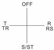
TVS33-□□ AS(3Ø3W 2CT) VS(3Ø3W)
