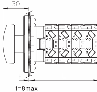
TVS33-□□ VS(3Ø3W)
